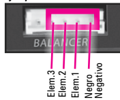
Ejemplo Conexión 3S:
