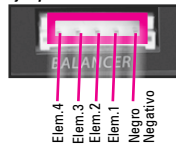
Ejemplo Conexión 4S:
