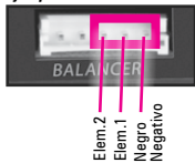
Ejemplo Conexión 2S:
