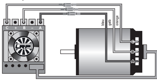
Hall-Sensor Anschlusskabel
