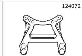
Dämpferbrücke vorne - S10 Twister TX, SC Front Shock Tower - S10 Twister TX, SC
