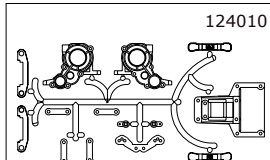
Getriebegehäuse - hintere Schwingenhalter Plastikteile - S10 Twister Gear Box - Rear Suspension Arm Hinge Pin Braces Plastics - S10 Twister
